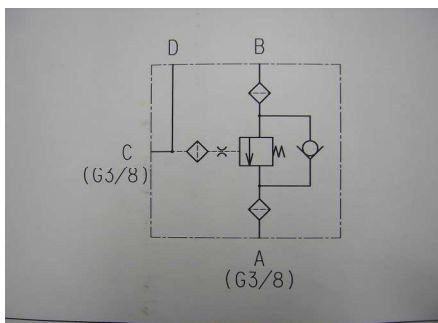
マニホールド(シングル)込み 回路図
