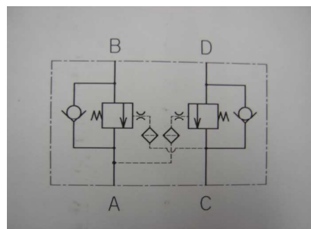
マニホールド(ダブル)込み 回路図
